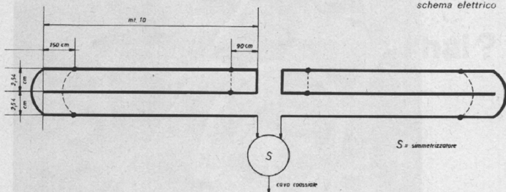
schema elettrico
