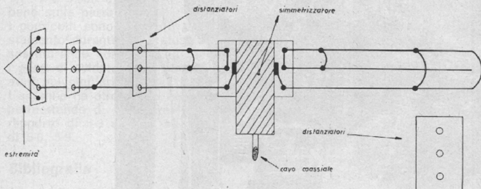
montaggio pratico
